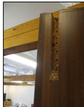
Voids in a fire door
